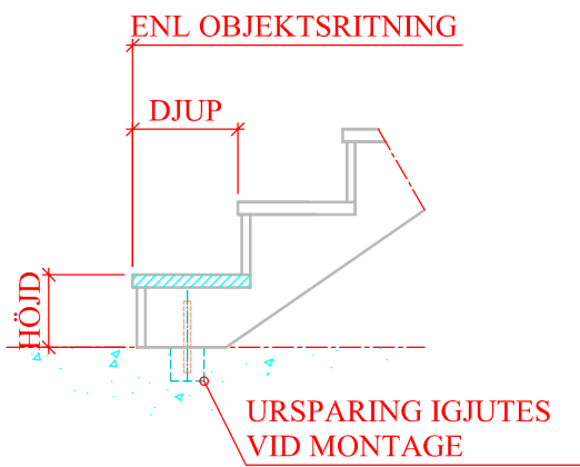
BÖRJAN FRÅN BOTTENPLATTA
