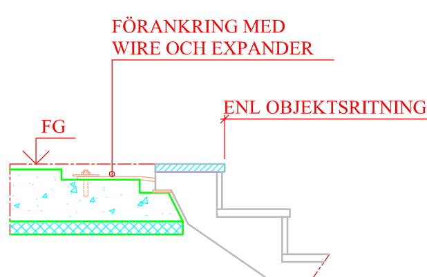
ANSLUTNING MOT BJÄLKLAG (EFTERMONTAGE)
