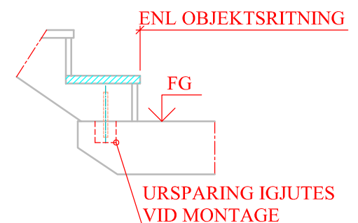
ANSLUTNING FRÅN VILPLAN
