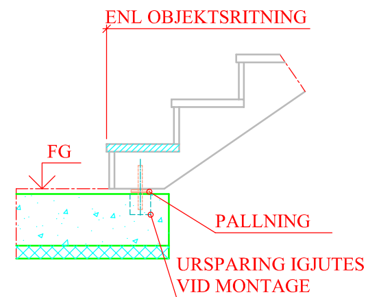
BÖRJAN FRÅN BJÄLKLAG
