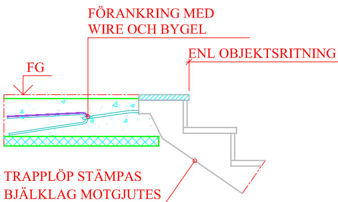
ANSLUTNING MOT BJÄLKLAG (MOTGJUTNING)
