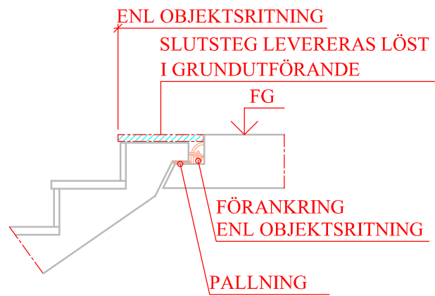
ANSLUTNING MOT VILPLAN
